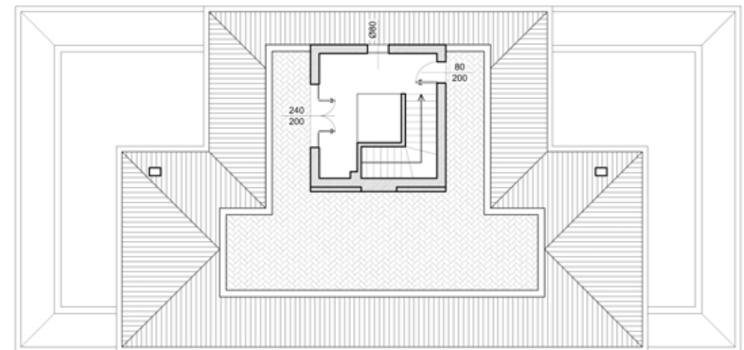
Copertura
