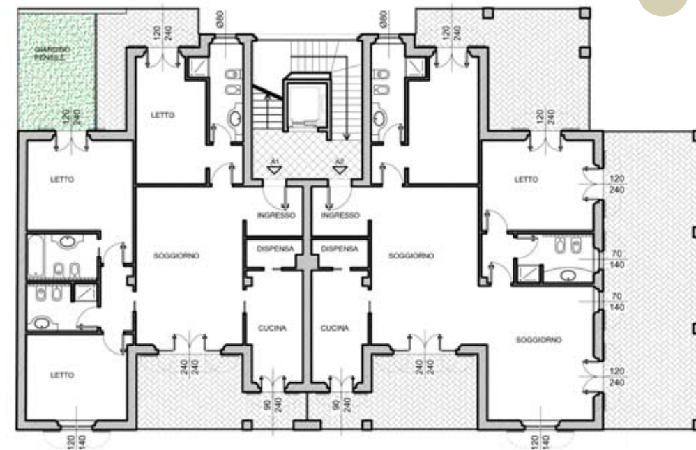
Primo Piano
