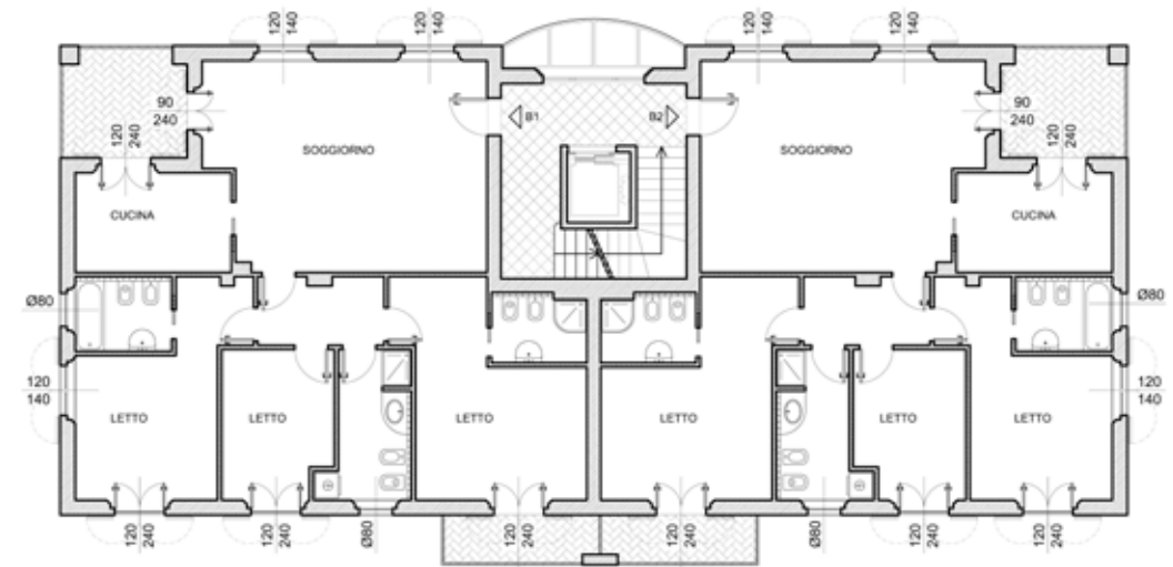
Primo Piano
